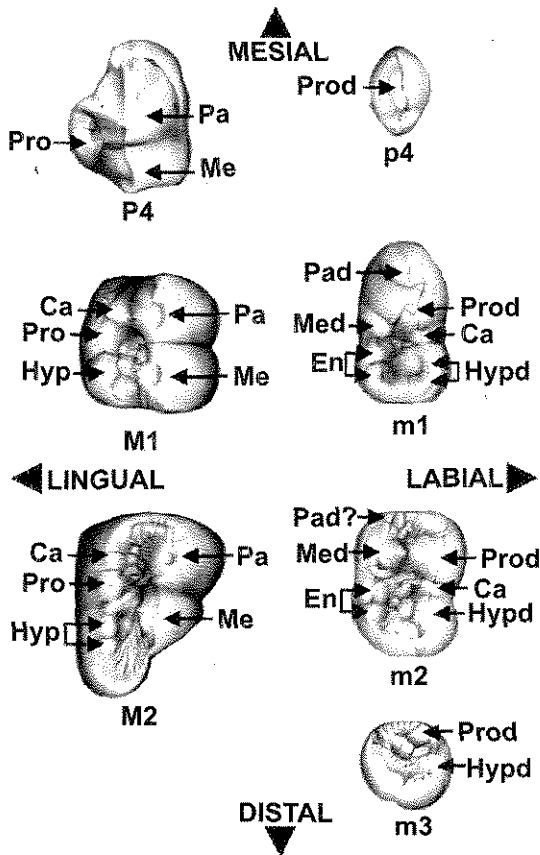
Fig. 1. Cúspides principales presentes en las series P4-M2 y p4-m3. Ca, cúspides accesorias; En, entocono; Hyp, hipocono; Hypd, hypoconido; Me, metacono; Med, metacónido; Pa, paracono; Pad, paracónido; Pro, protocono; Prod, protocónido. Nomenclatura de Torres (1988).
